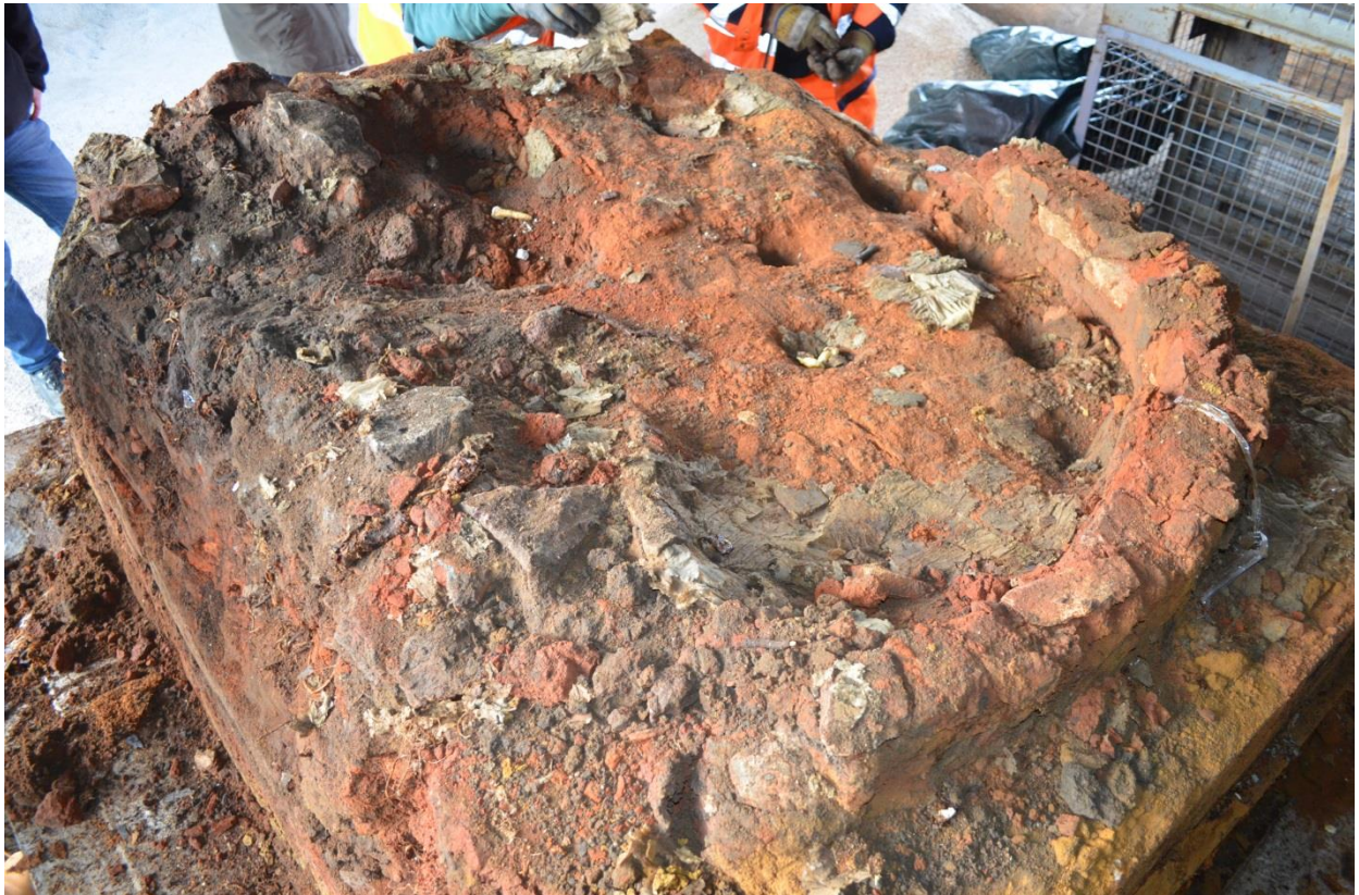
Abbildung 2: blockgeborgener Töpferofen nach der Entfernung der Einhausung
